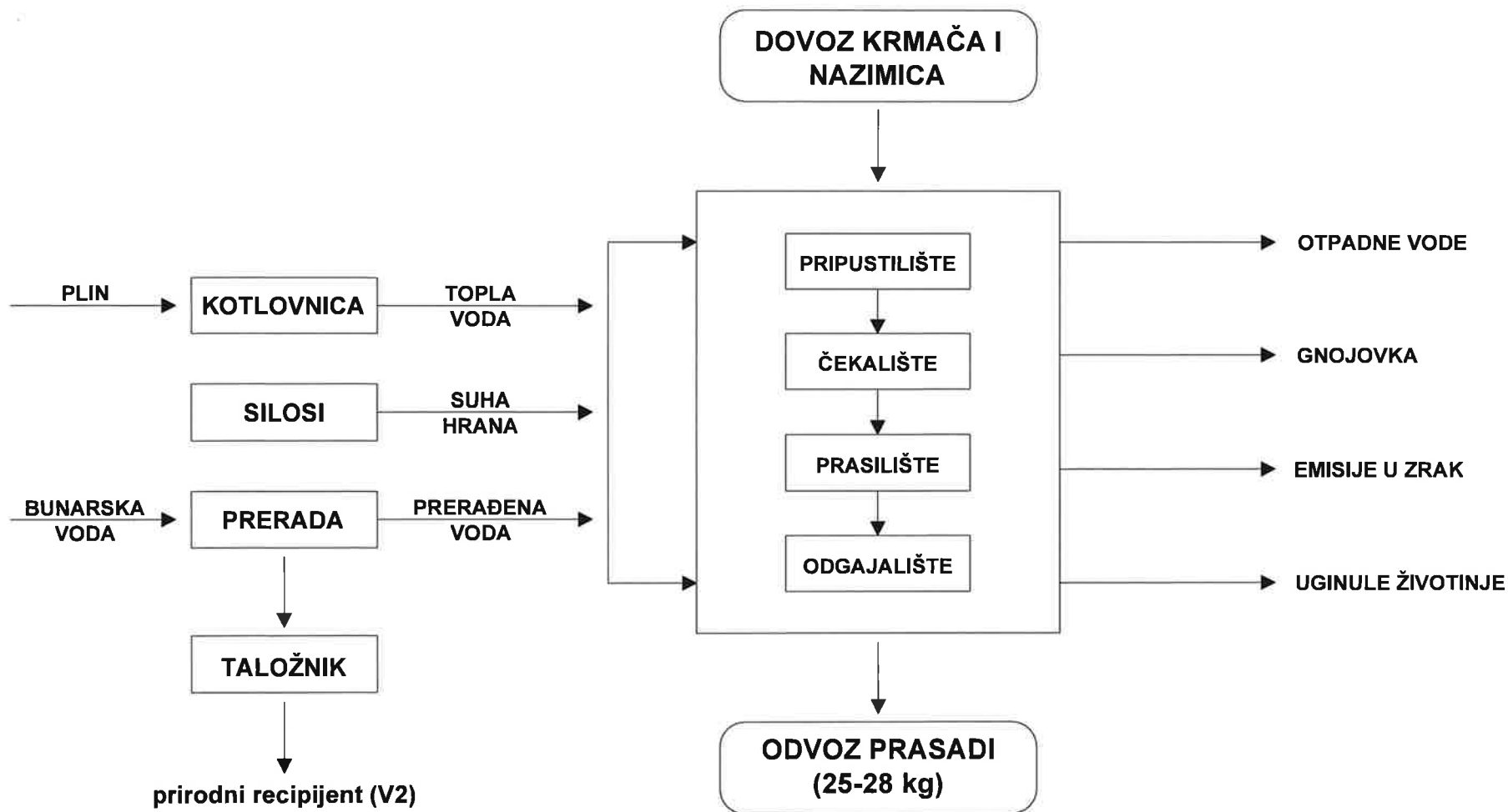
Prilog 2. Blok dijagram tehnološkog procesa na Farmi svinja Gaj
